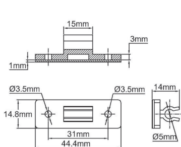
Kolbenhalterung, gestanzter Stahl, für Kolben Ø 5-6mm
